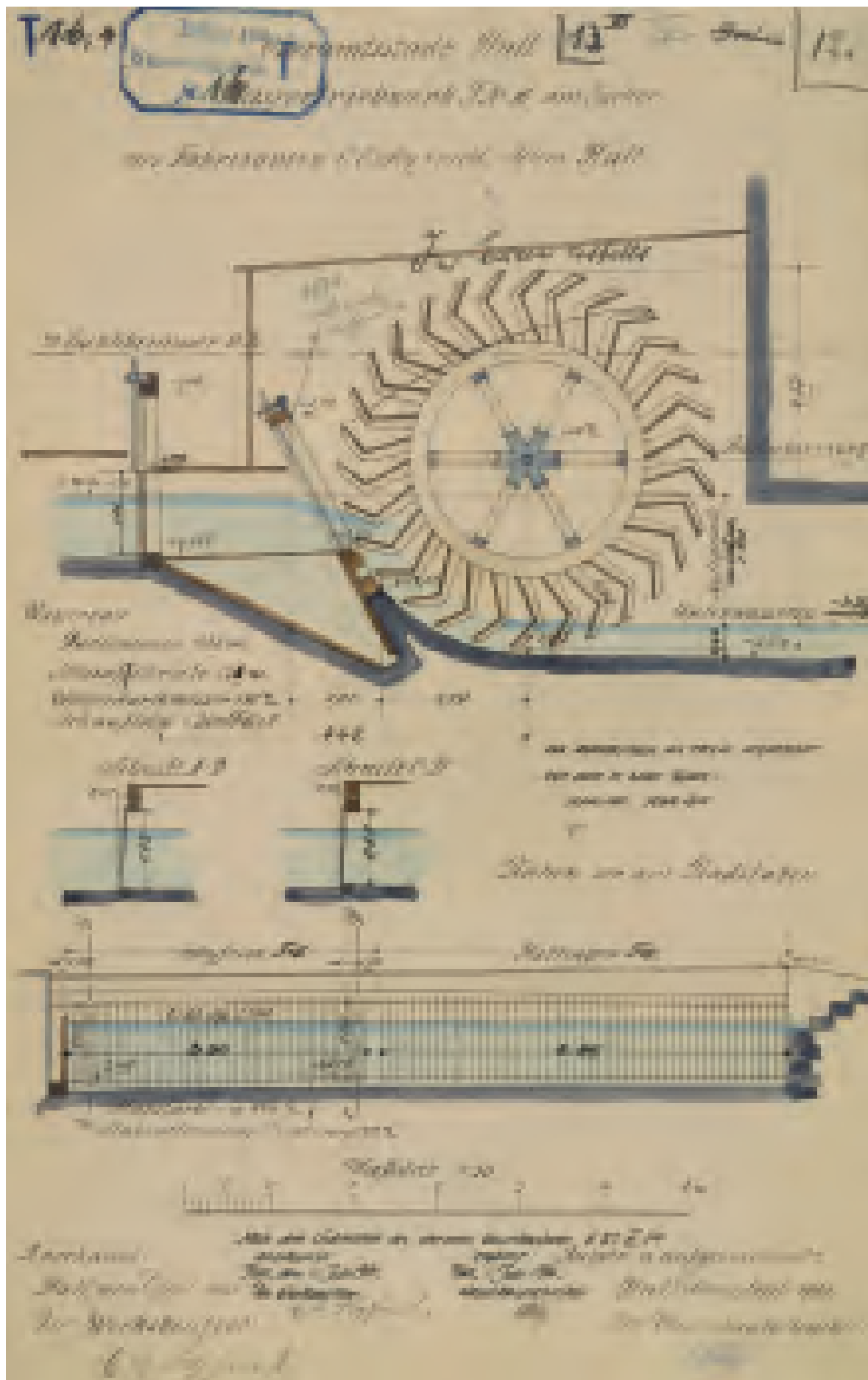
Wassertriebwerk des Fabrikanten C. E. Seyfried am Kocher in Schwäbisch Hall von 1913 aus den Triebwerksakten zu den Wasserbüchern. Vorlage: Landesarchiv StAL EL 20/6 II Bü. 60 Qu. 12
